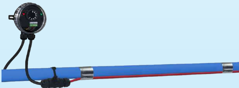
Esempio di montaggio su un cavo di tracciamento del calore, con scatola di connessione Y24, per la protezione antigelo di tubi in PVC
